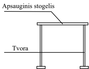
TVOROS SU APSAUGINIU STOGELIU ĮRENGIMO FRAGMENTAS
